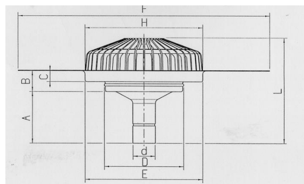
Fig. 1: Coupe verticale à travers l'avaloir de toiture
