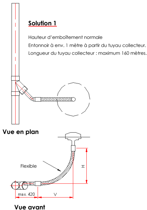
Fig. 2: Avoir et tuyau collecteur
